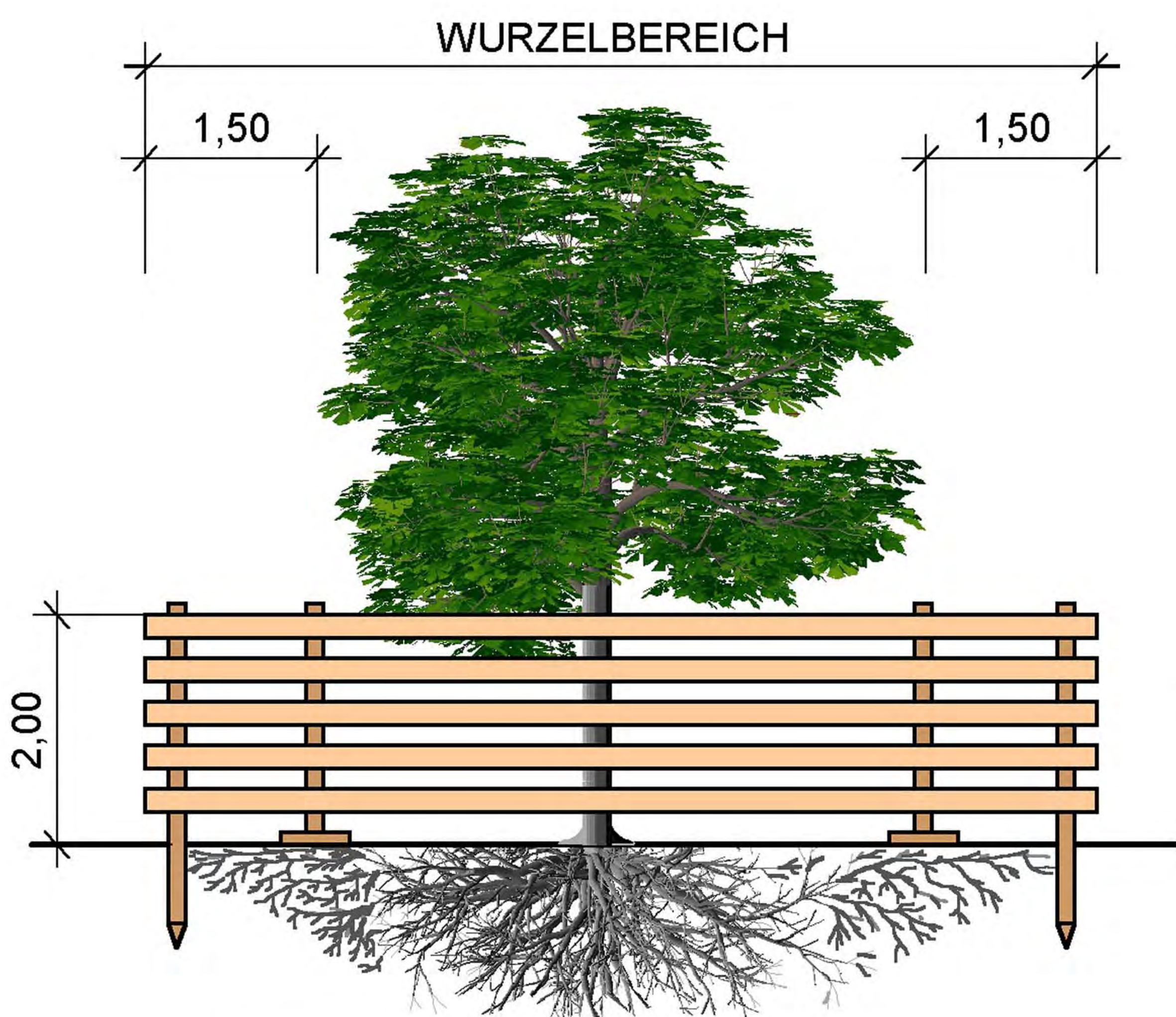
WURZELSCHUTZ DURCH ZAUN
